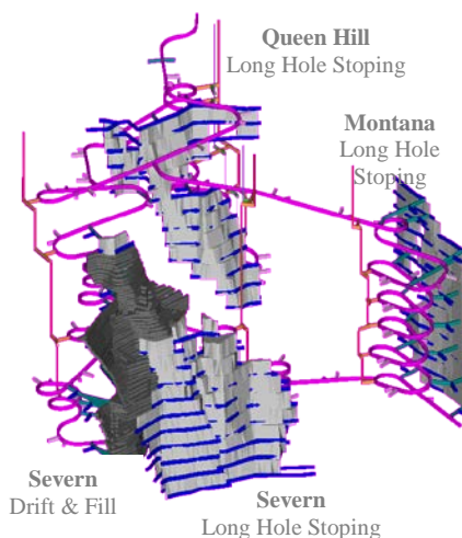
ホームスケルク地下鉱山計画
